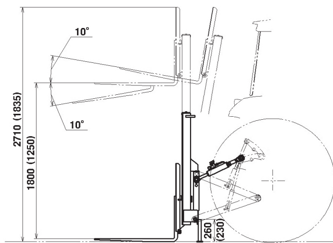
仕様図
