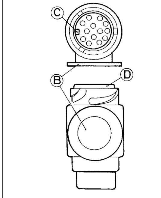
トレーラコンセントオス詳細
